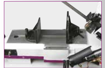
Schnellspannschraubstock › Verstellbare Spannbacken von 0° bis 45° für Gehrungsschnitte
